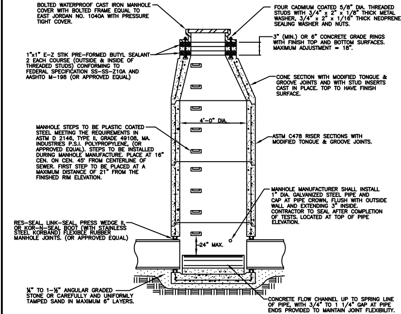
STANDARD MANHOLE
